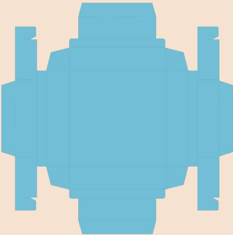
抽屉式盒型 105*105*27mm
